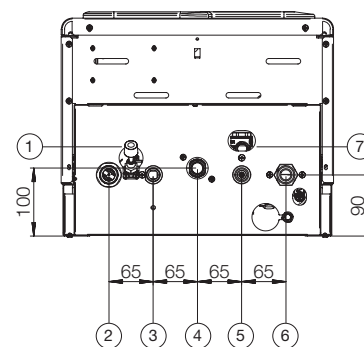
Vista inferior
